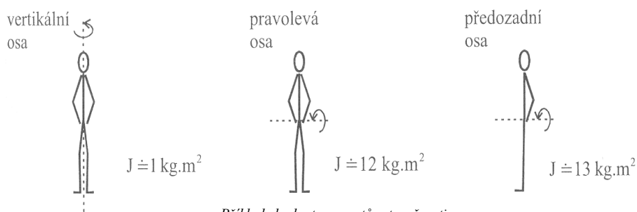
Příklady hodnot momentů setrvačnosti.
